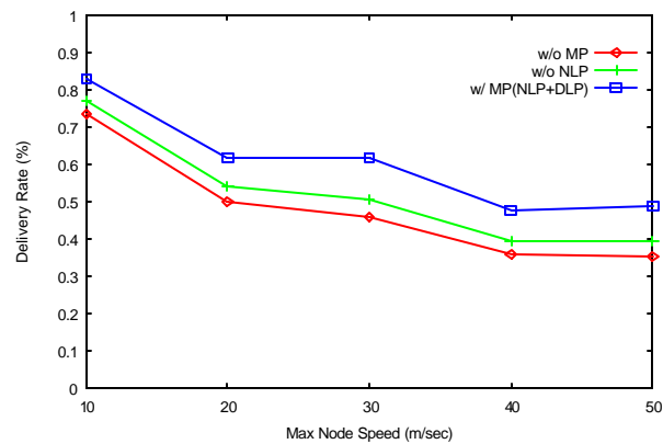
(d) SDR under RPGM
